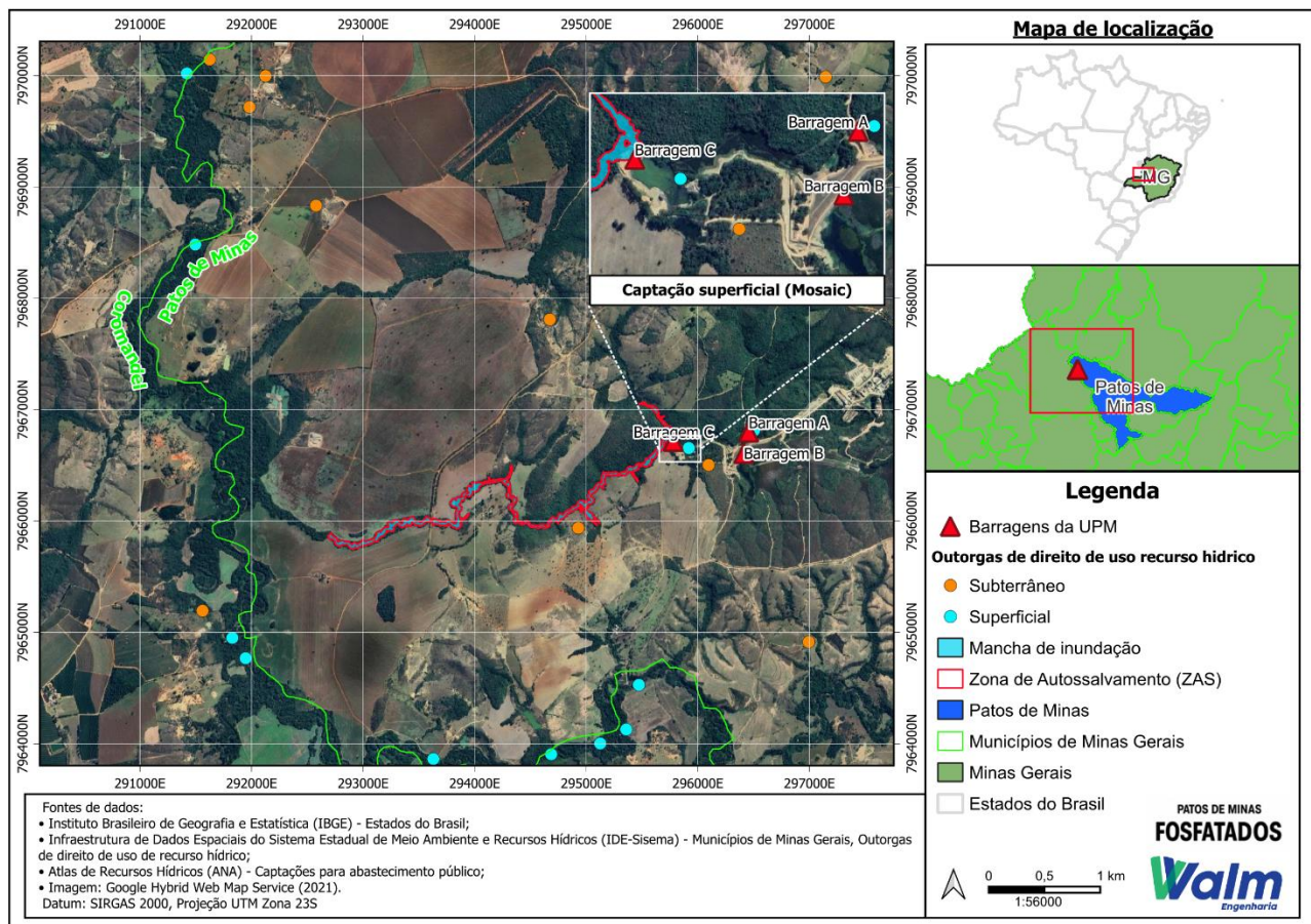
Figura 2 - Outorgas de direito de uso de recurso hídrico identificadas nas proximidades da Barragem C, com detalhe para a captação superficial inserida na mancha
