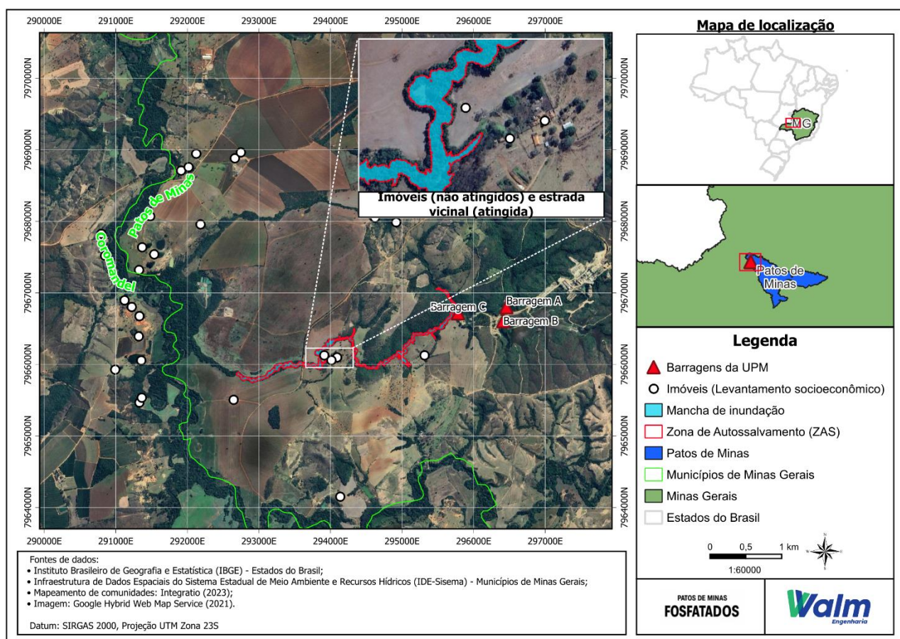
Figura 1 - Envoltória máxima de inundação da Barragem C
